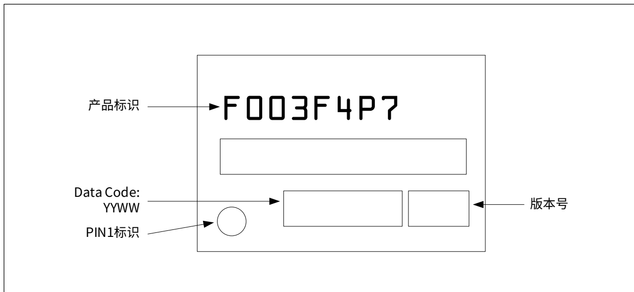
图 8-4 TSSOP20 顶部标记示例
