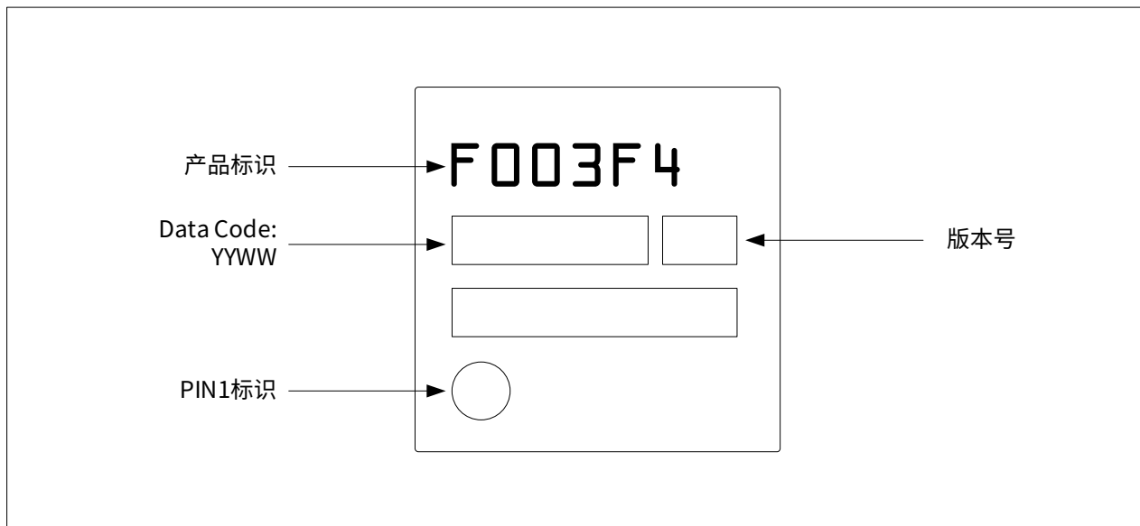
图 8-6 QFN20 顶部标记示例
