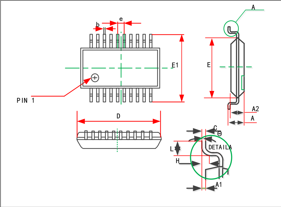
图12 TSSOP20 封装图
