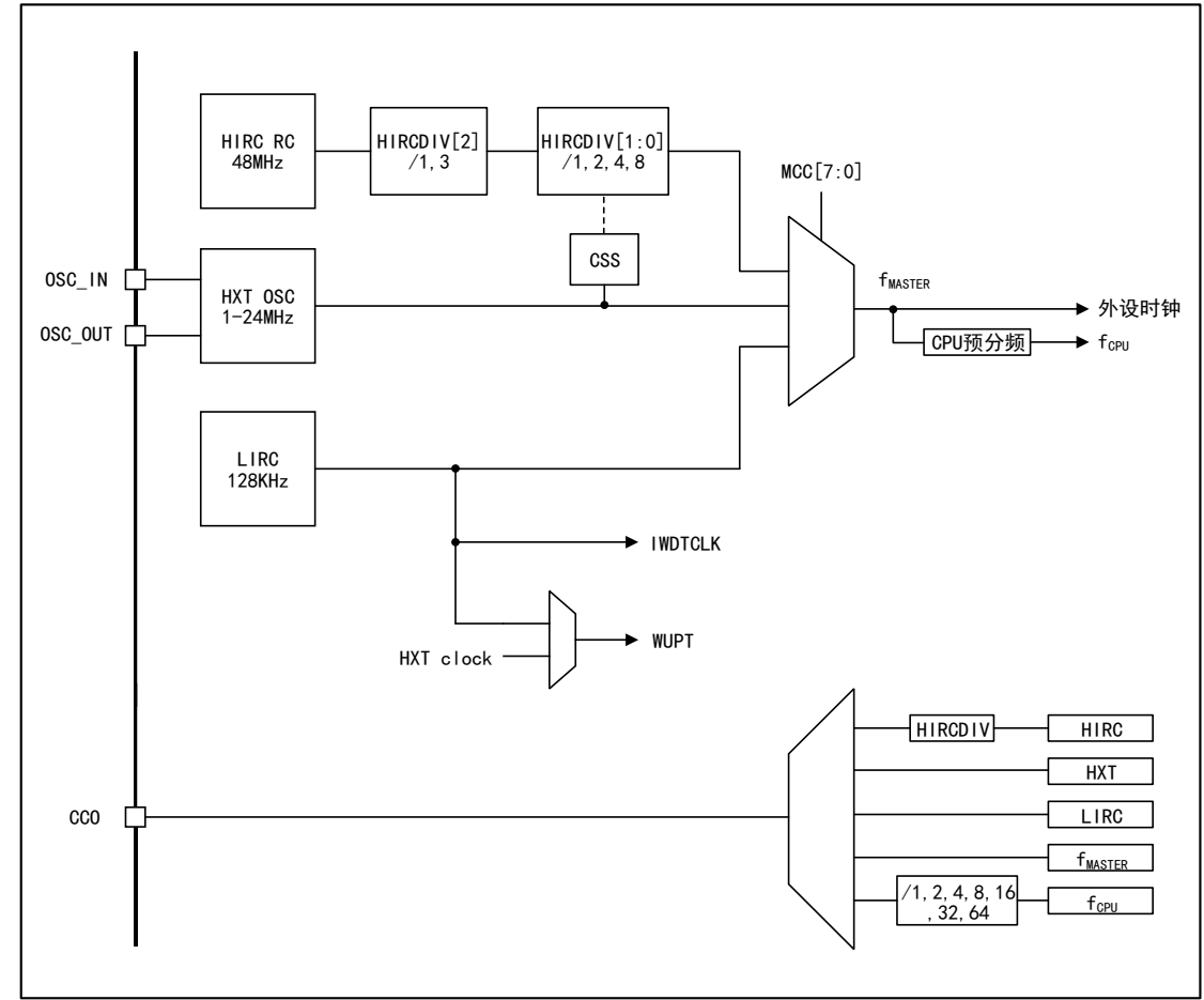
图5 APM32F003x4x6 系列时钟树
