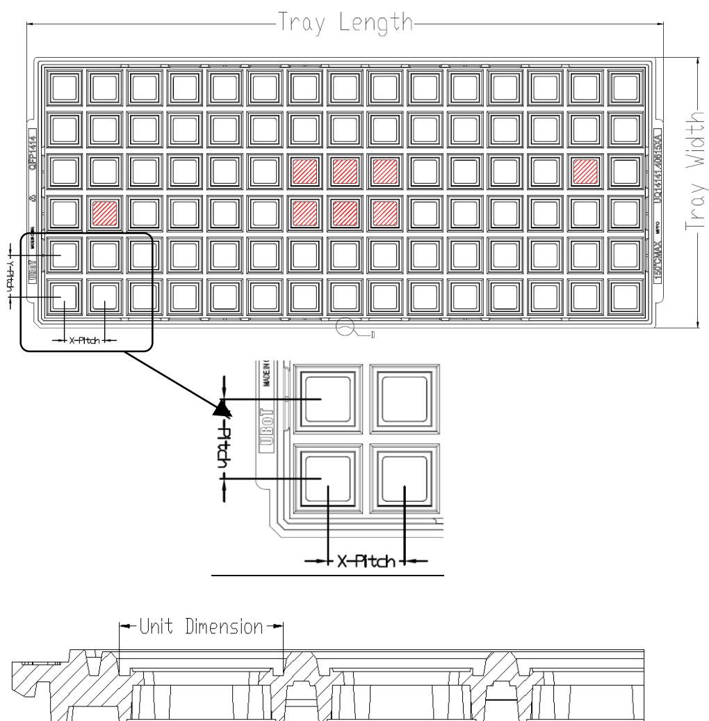
图19 纸盘尺寸
