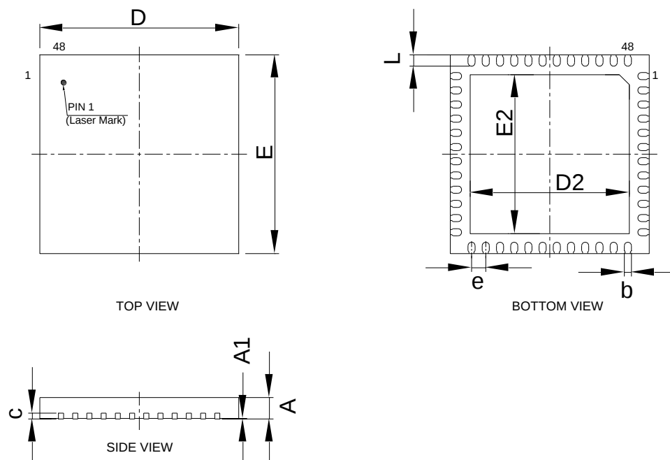
图 25 QFN48 封装图
