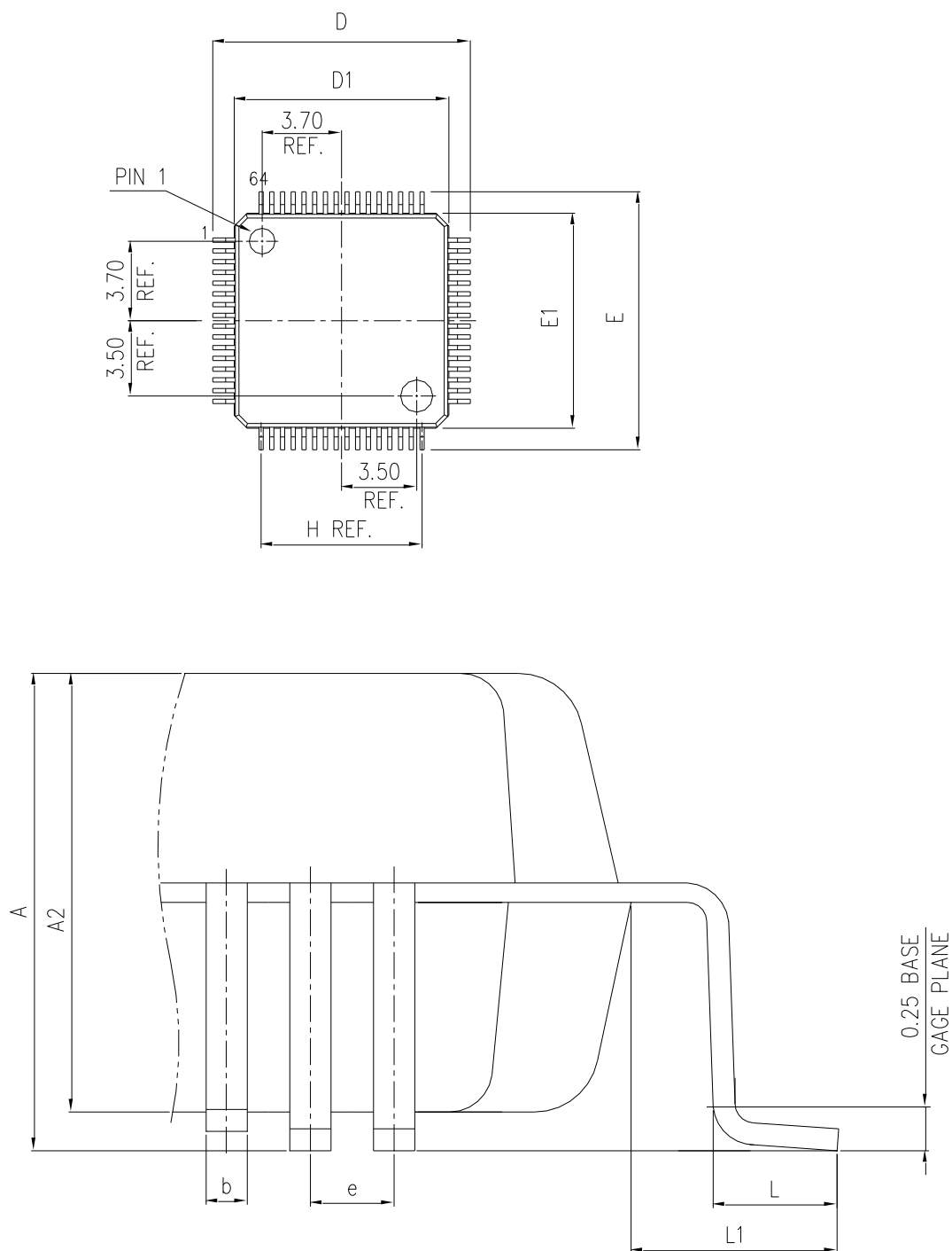
图 19 LQFP64 封装图
