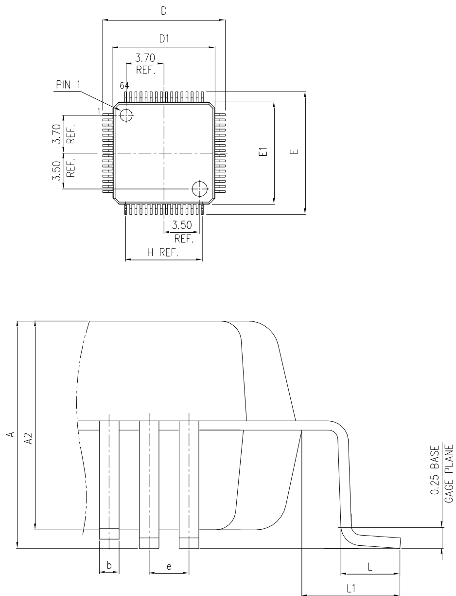
图 19 LQFP64 封装图
