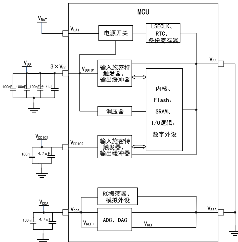
图 7 电源方案
