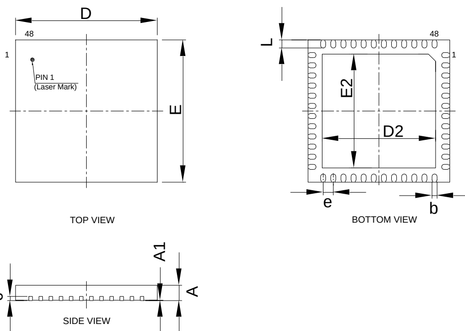
图 25 QFN48 封装图
