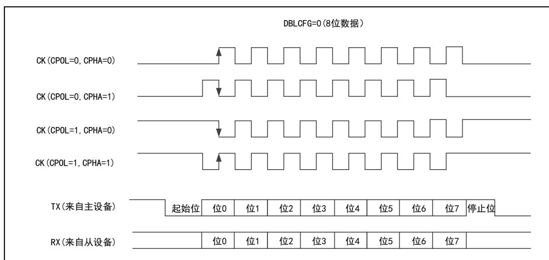
图 67 USART 同步传输时序图 (DBLCFG=0)
