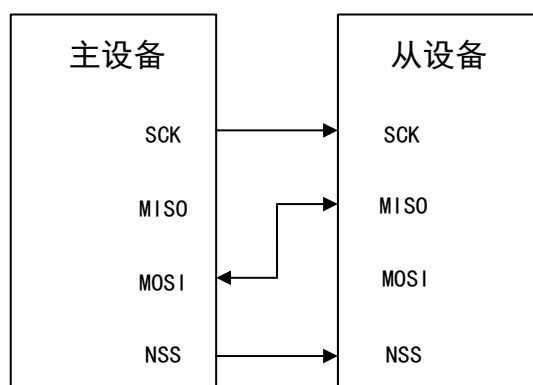
图 86 双向线连接
