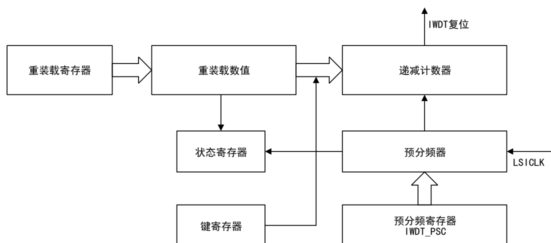
图 60 独立看门狗结构框图
