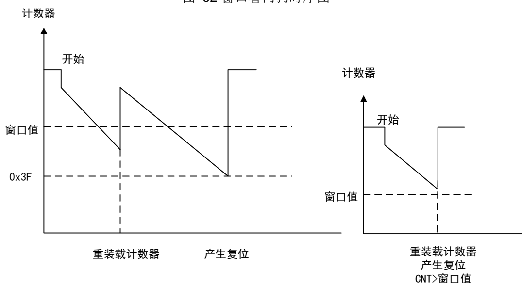
图 62 窗口看门狗时序图
