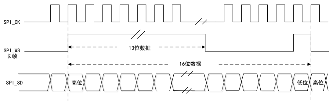
图 96 PCM 标准波形
