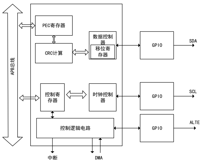
图 75 I2C 功能结构图
