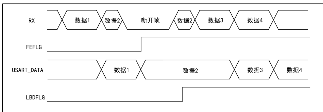
图 70 数据传输状态检测断开帧
