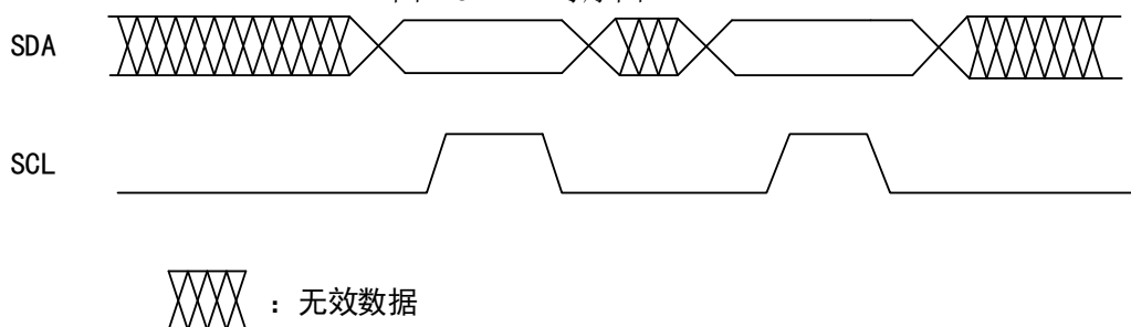
图 79 SDA 时序图
