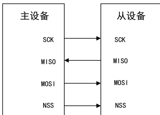
图 83 全双工模式连接
