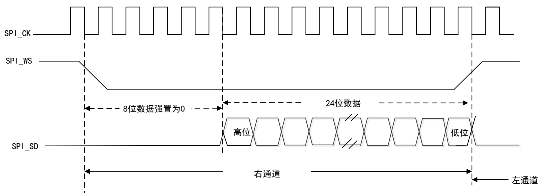
图 94 LSB 对齐标准波形（24 位数据）
