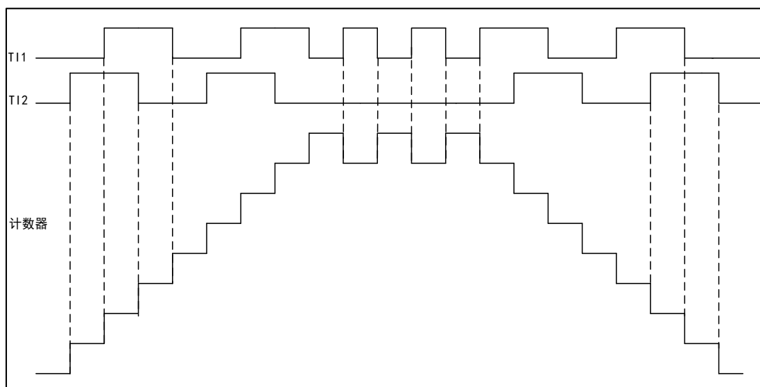
图 54 编码器模式下的计数器操作实例
