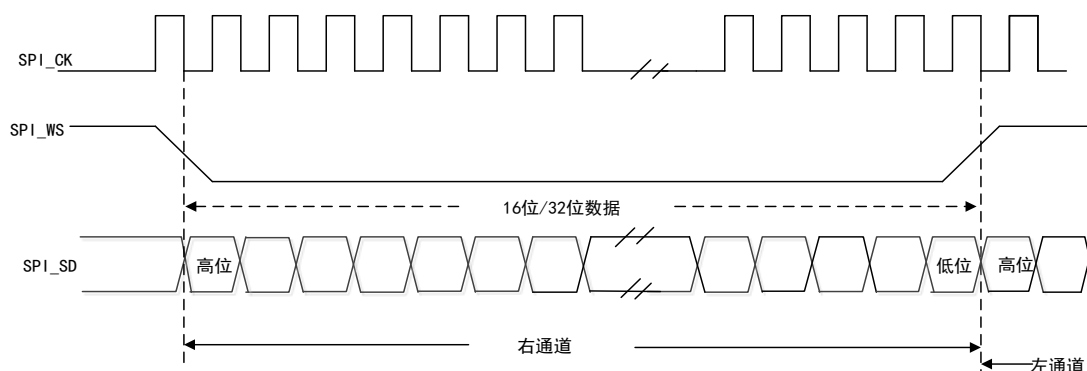
图 91 MSB 对齐标准波形（24 位数据）
