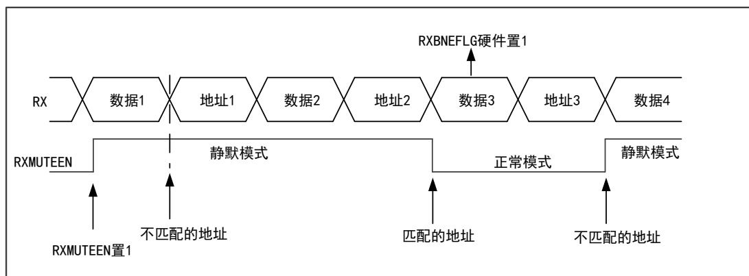
图 65 地址标记退出静默模式
