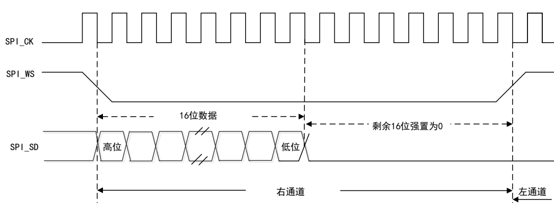
图 92 MSB 对齐标准波形（16 位扩展至 32 位）
