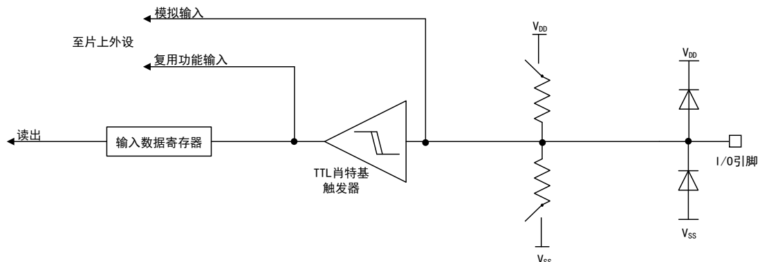
图 18 输入模式结构
